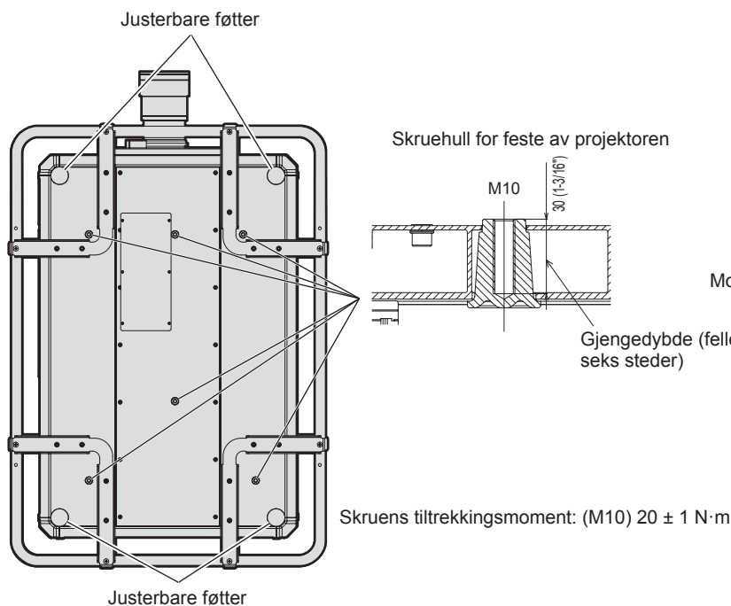
Skruehullenes posisjon for feste av projektor og justerbare føtter
