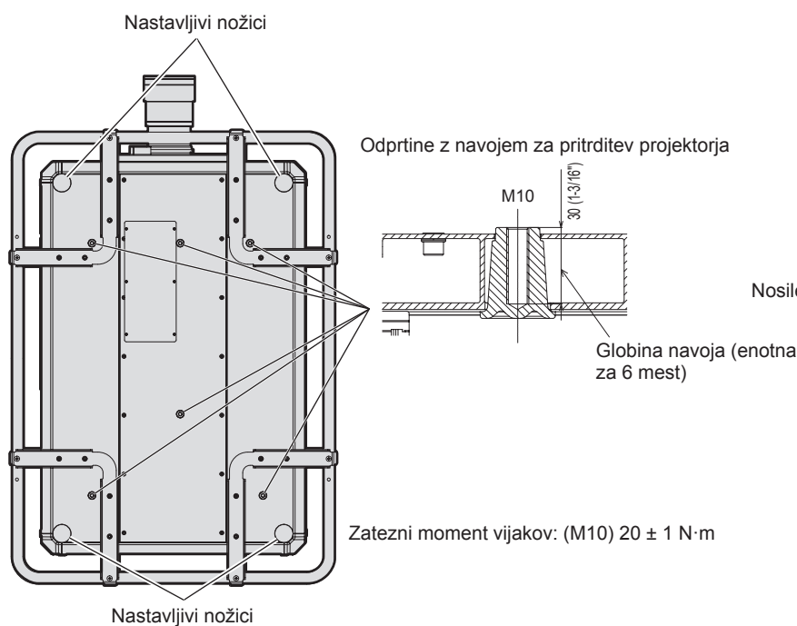
Mesta odprtini z navojem za pritrditev projektorja in nastavljive nožice
